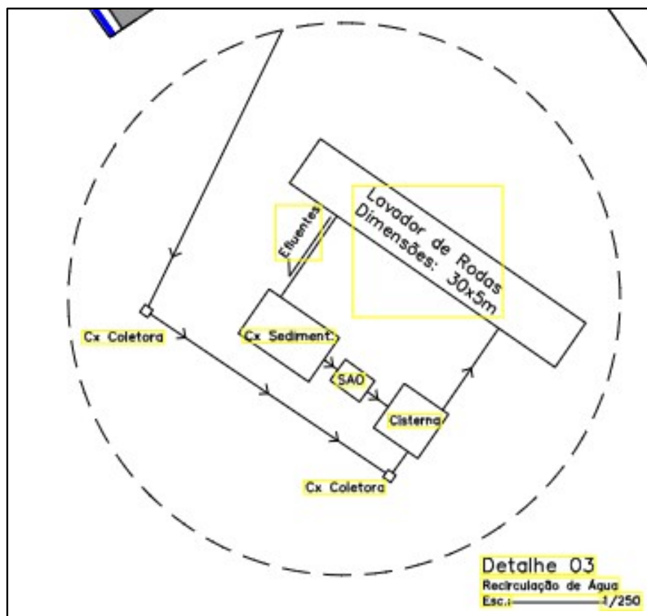
Figura 4 – Representação da área do Lava Pneu
